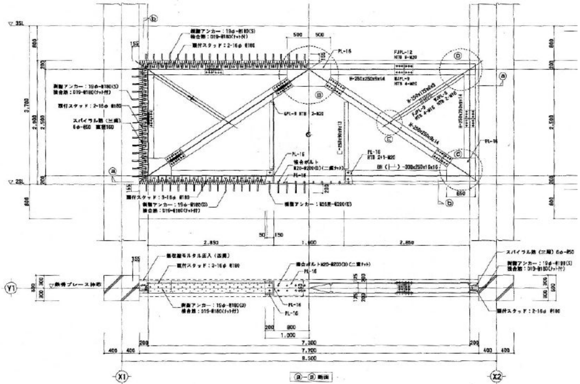
解図 3.4.6-6 鉄骨下枠切断K型ブレース詳細図
